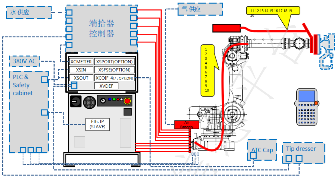
图2 机器人电缆配置图
