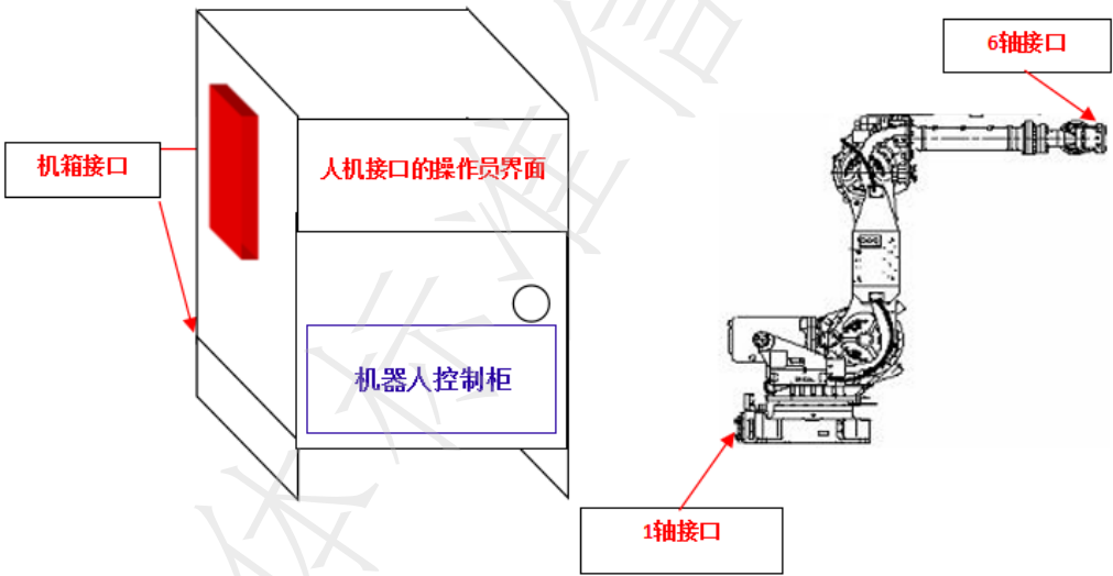
图1 机器人结构图
